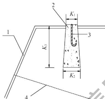
图 B.0.3-2 基坑边坡顶水平位移监测点
